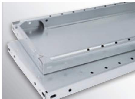
Stahlfachboden mit Rohrkante für höchste Stabilität und für optimale Benutzersicherheit sowie Systemlochung im Raster 50 mm für steckbares Zubehör
